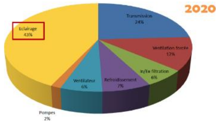
Consommation d'énergie primaire – bureaux Source / Bron : CSTC
