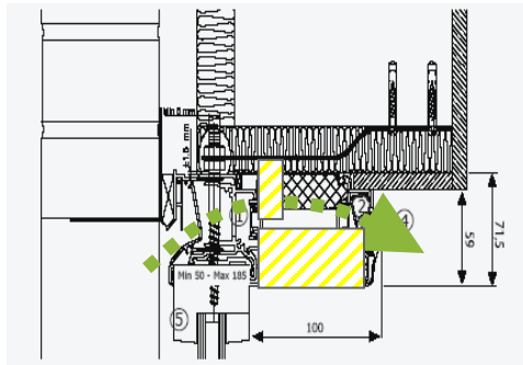
prise d'air réglable acoustique
