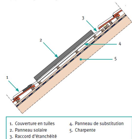
Fig. 9 Montage en semi-intégration.
