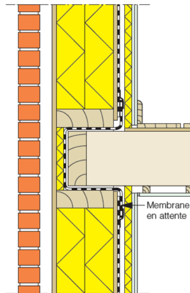
Raccord façade / plancher intermédiaire Source: Buildwise
