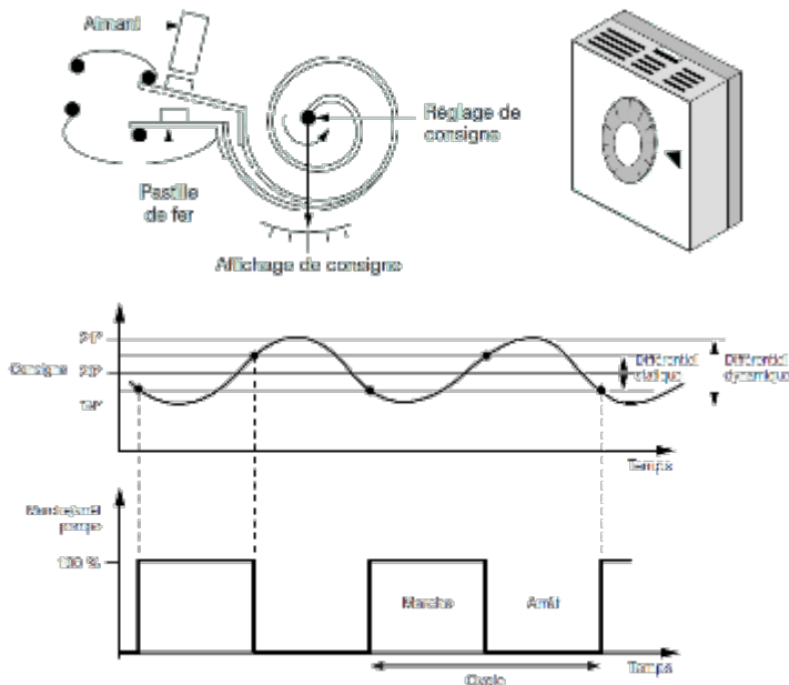
Fig. 42 Variation de température générée par un signal thermostat d'ambiance maitrisé.
