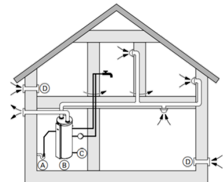
Représentation système pour une utilisation sur air évacué
