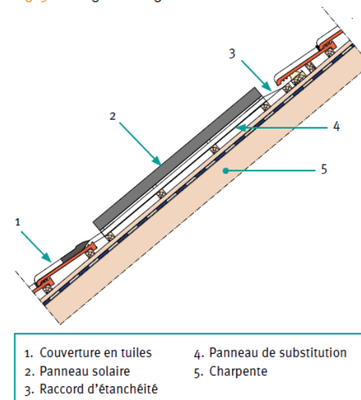
Fig. 9 Montage en semi-intégration.
