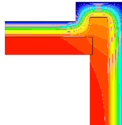
Coupe – flux thermiques
