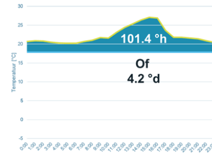
Zomerdag - Koelvraag
