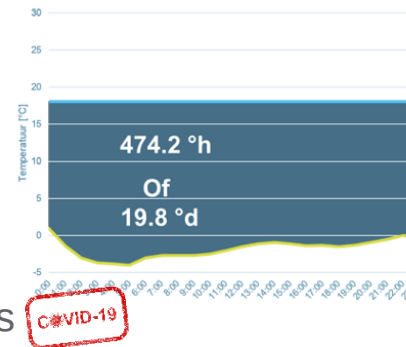
Winterdag - Warmtevraag
