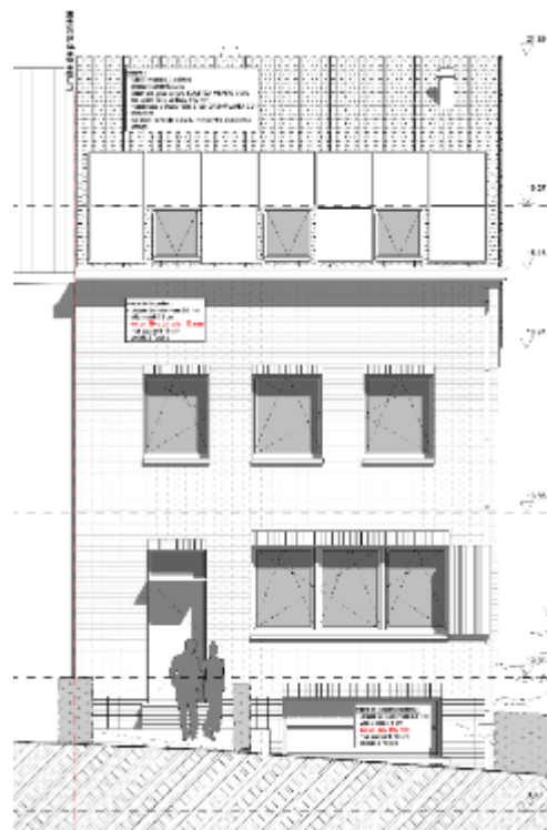
Elévation – Projet – APRES Isolation par l'extérieur
