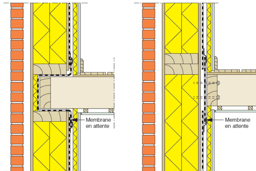
Raccord façade / plancher intermédiaire Source: Buildwise
