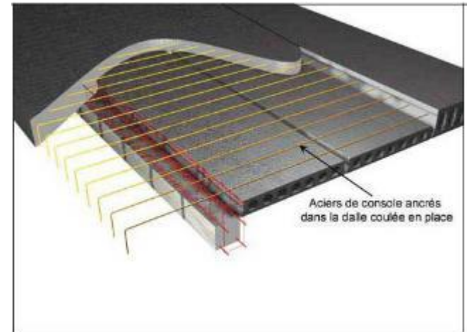
Dalle de compression Source : SEAC
