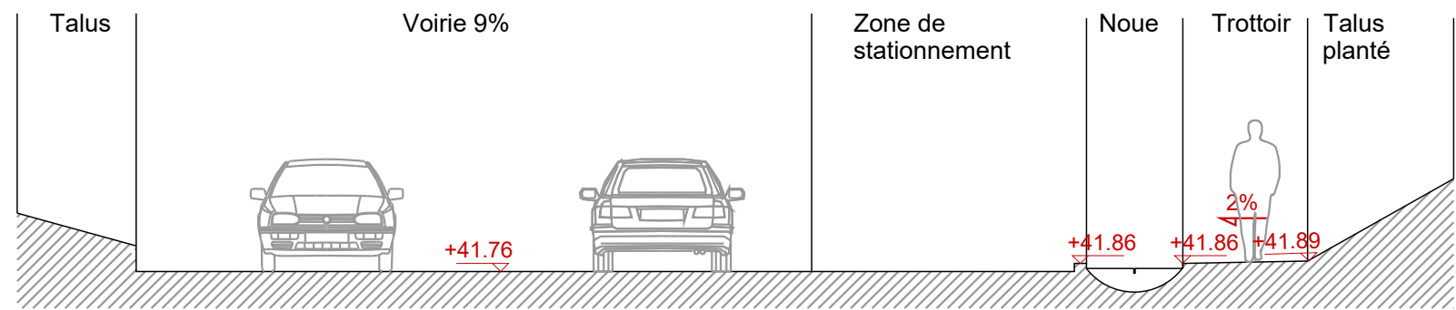
Profil 1_voirie à 9%
