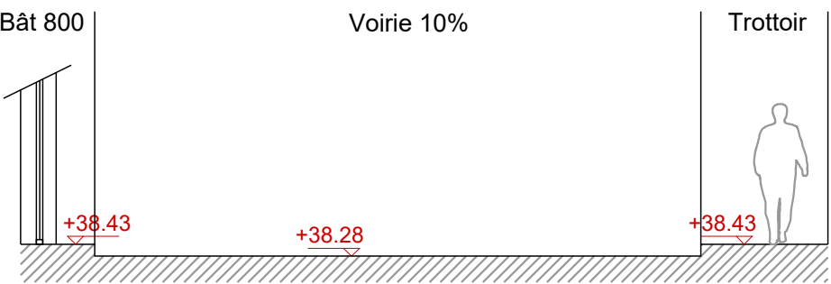
Profil 4_voirie à 10%
