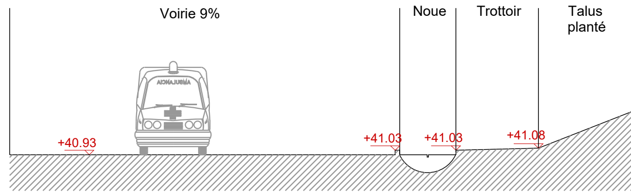
Profil 2_voirie à 9%
